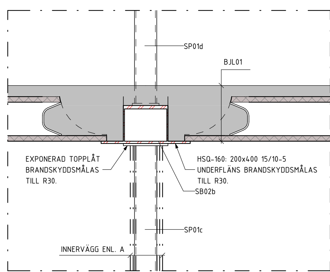
D - D 1 : 10
