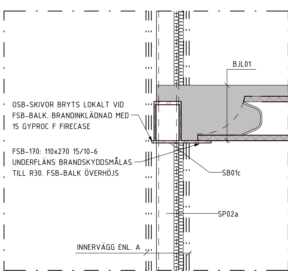
C - C 1 : 10
