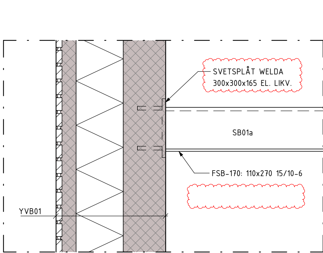
A - A 1 : 10
