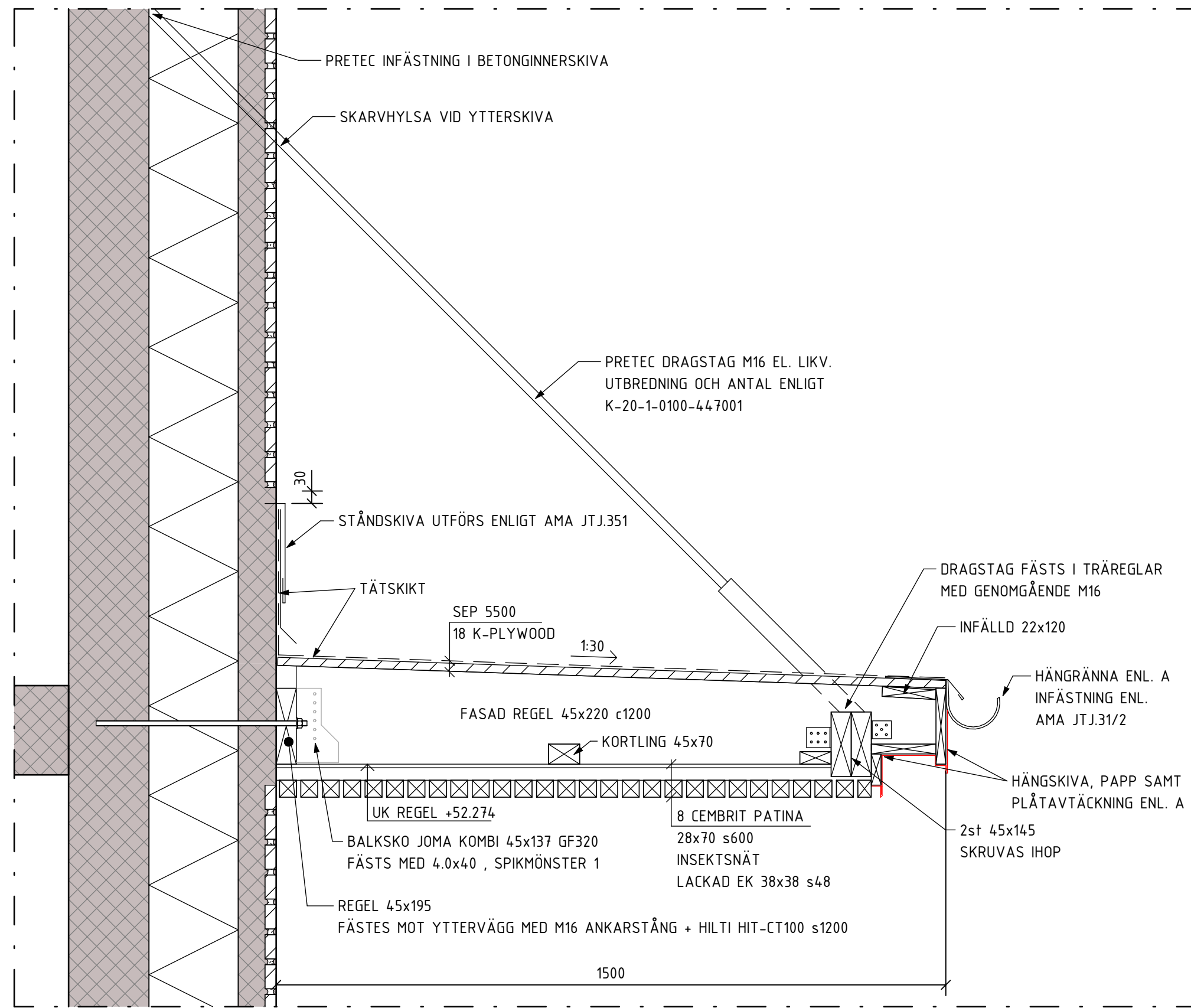
H - H 1 : 10
