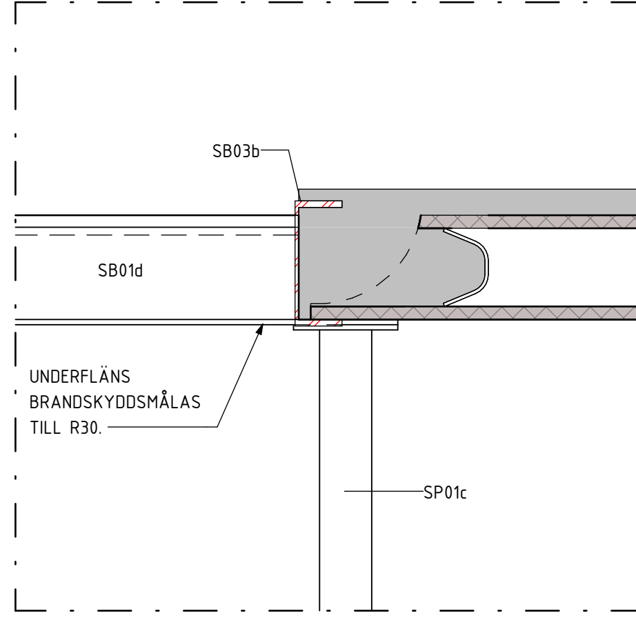
G - G 1 : 10
