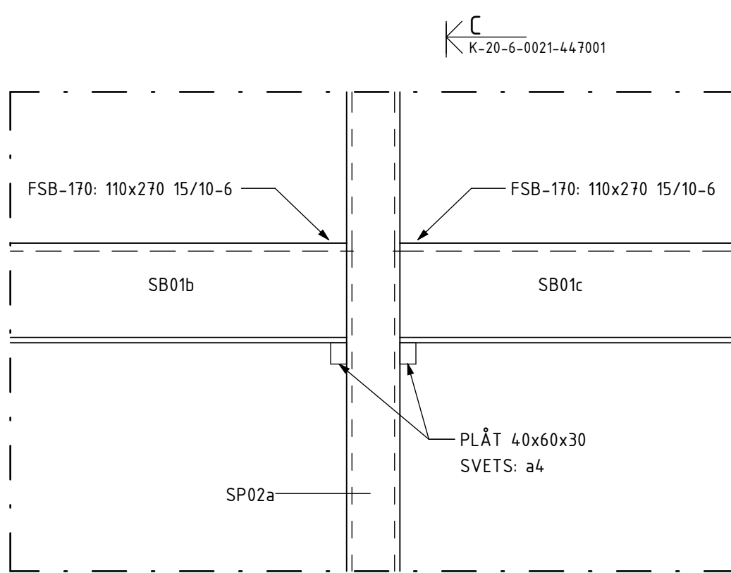
B - B 1 : 10
