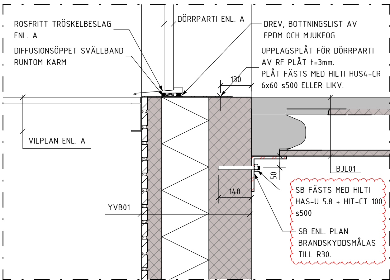
E - E 1 : 10
